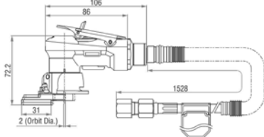
Mit Schleifplatte, 26 x 50 mm With rectangular pad, 26 x 50 mm
